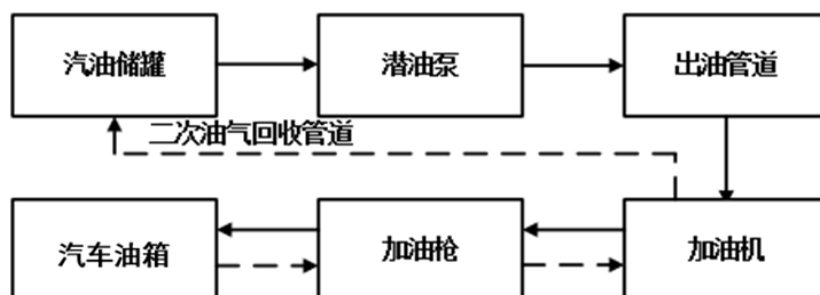
图 2.6-3 汽油加油流程图
