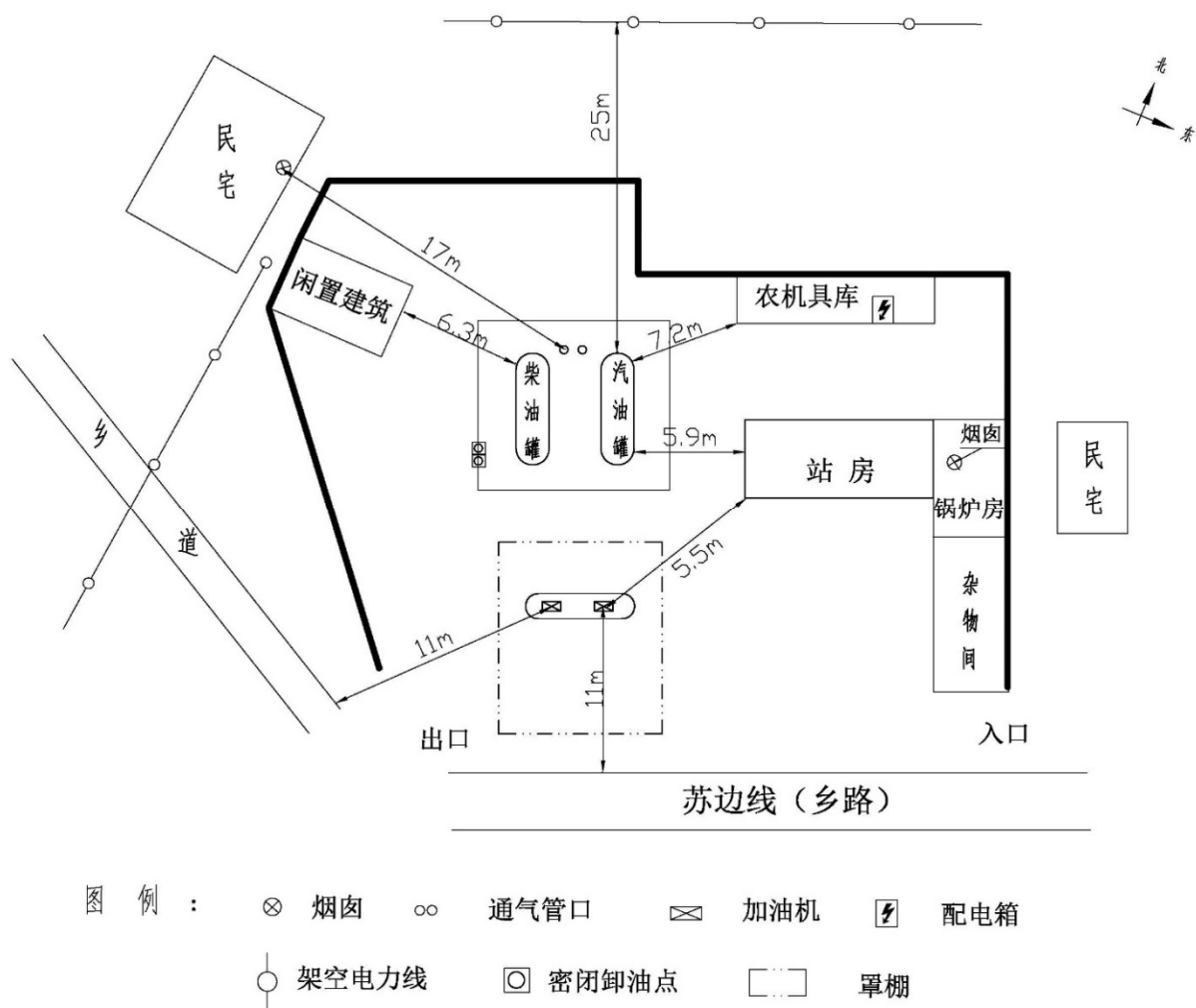
图 2.3-1 加油站总平面布置图
