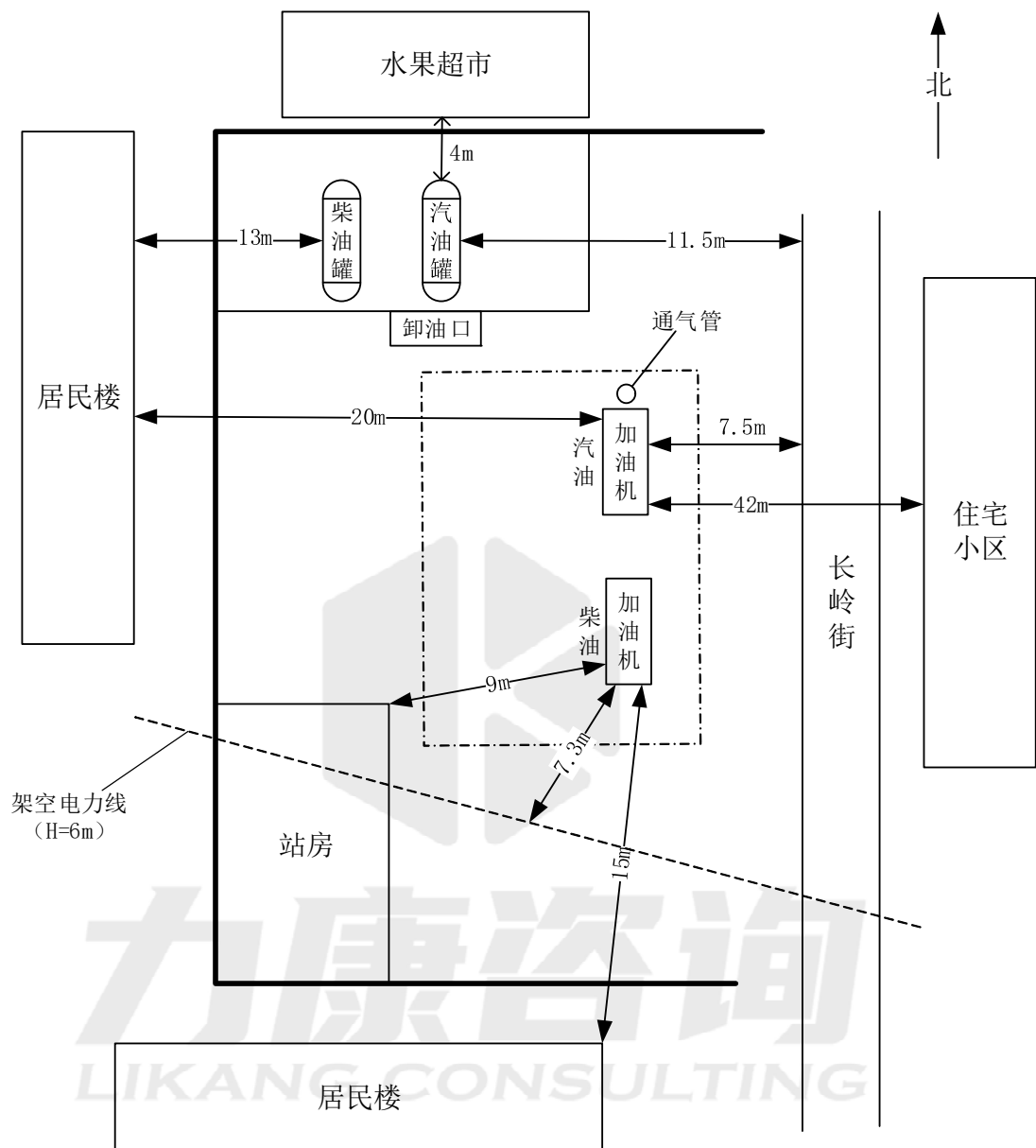
图 2.3-1 加油站总平面布置图
