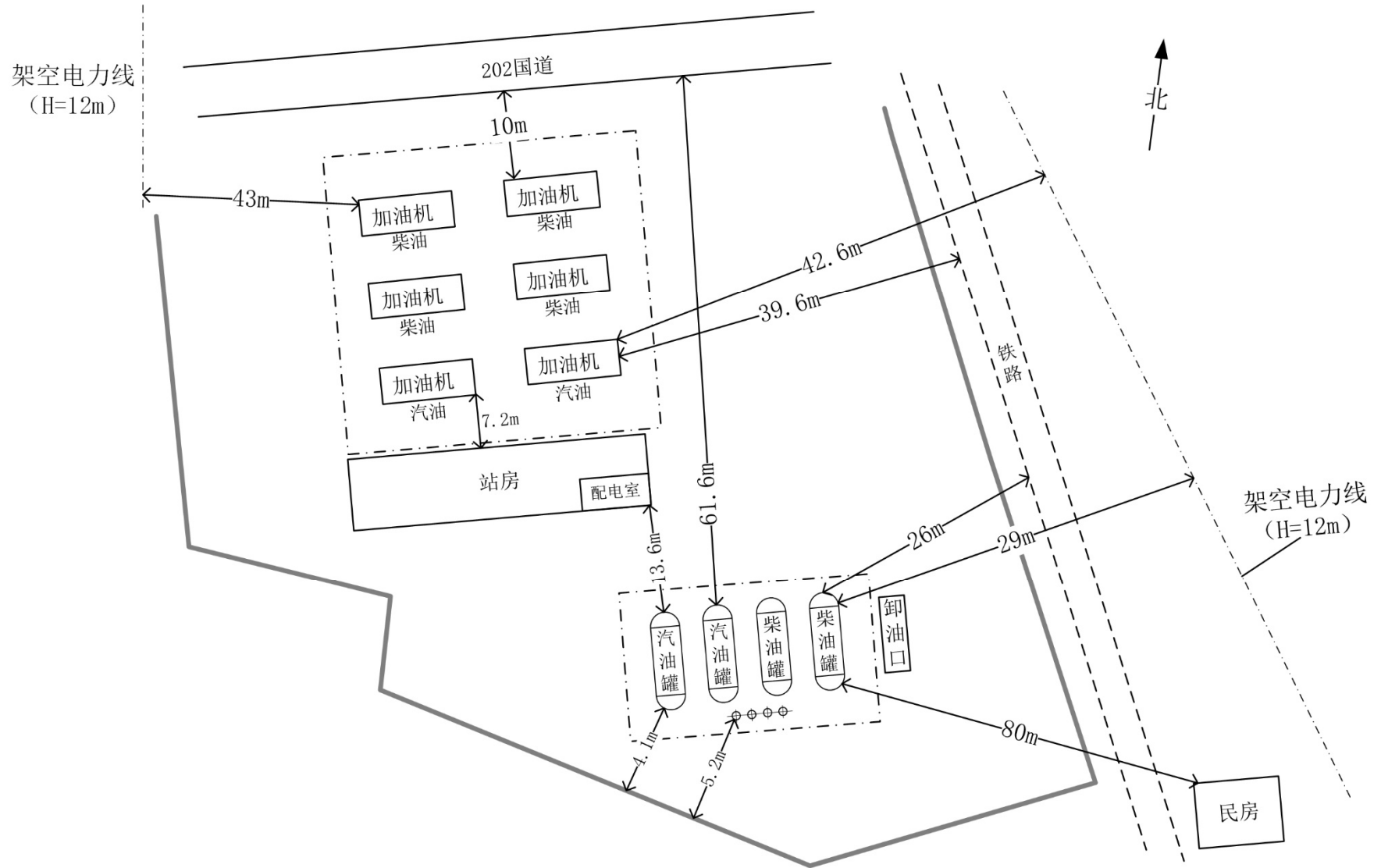
图 2.3-1 加油站总平面布置示意图
