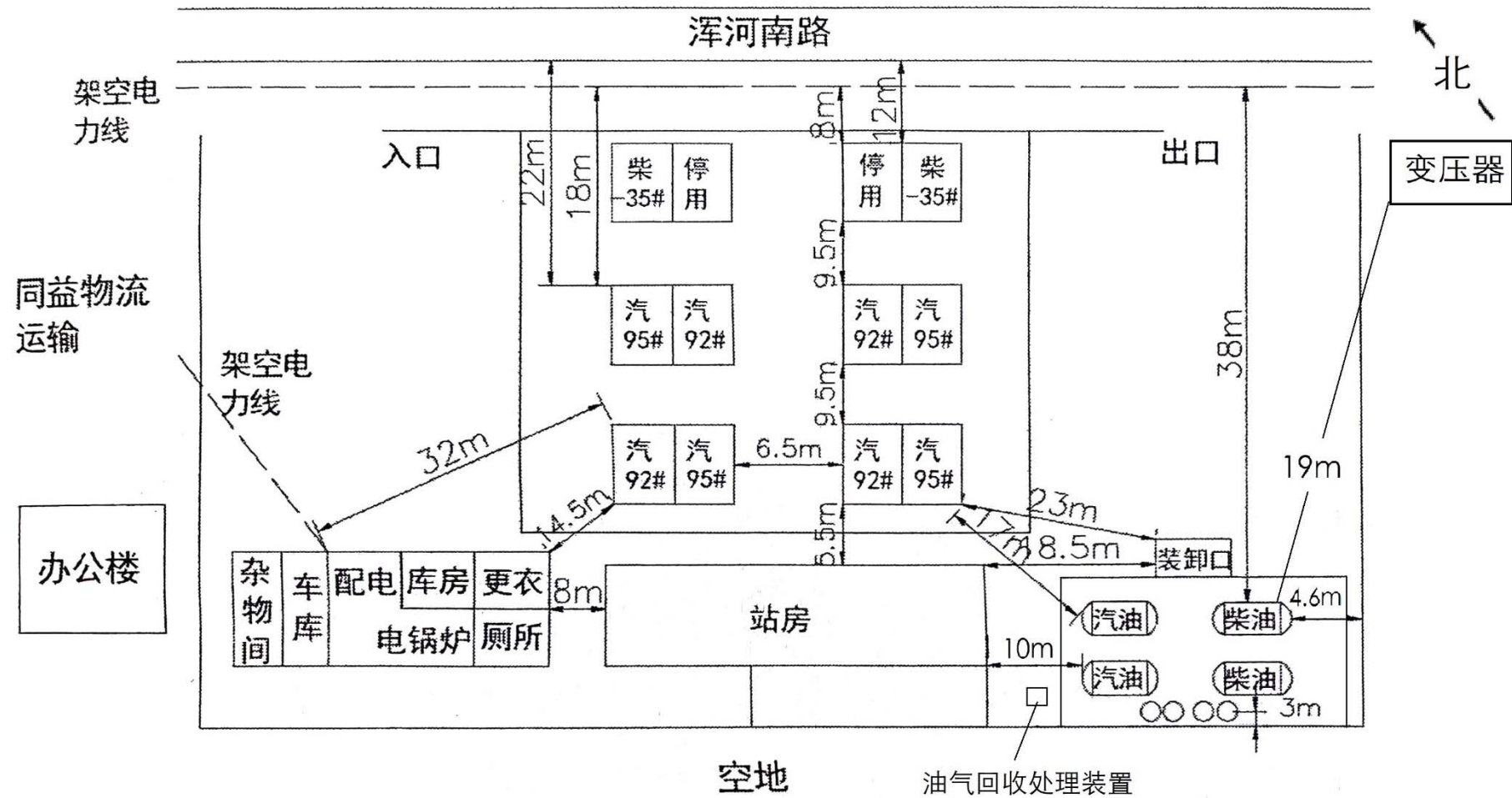
图 2.3-1 加油站总平面布置示意图
