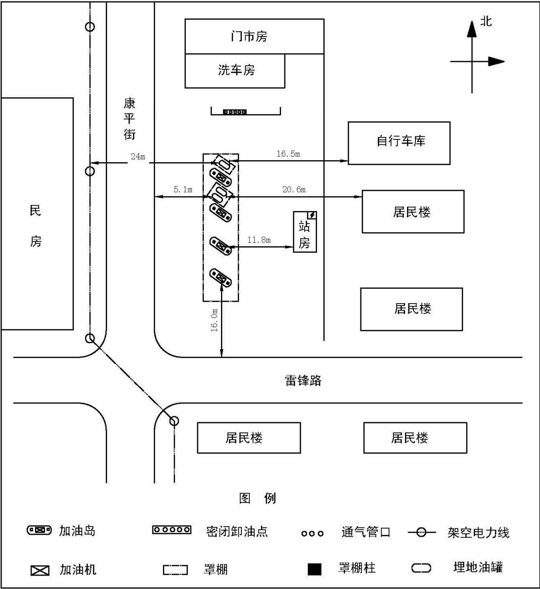
图 2.3-1 总平面布置示意图
