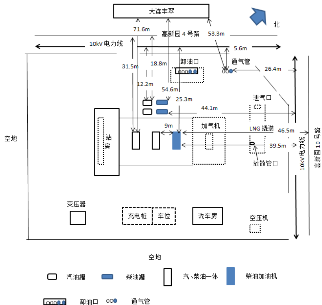
图 2.4-2 项目平面布置及周边环境示意图（图中实线部分为该项目评价范围）
