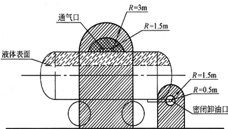
图 6.3-2 油罐车卸车用乙醇汽油时爆炸危险区域划分
