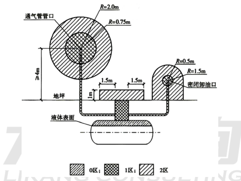
图 6.3-3 埋地卧式车用乙醇汽油储罐爆炸危险区域划分
