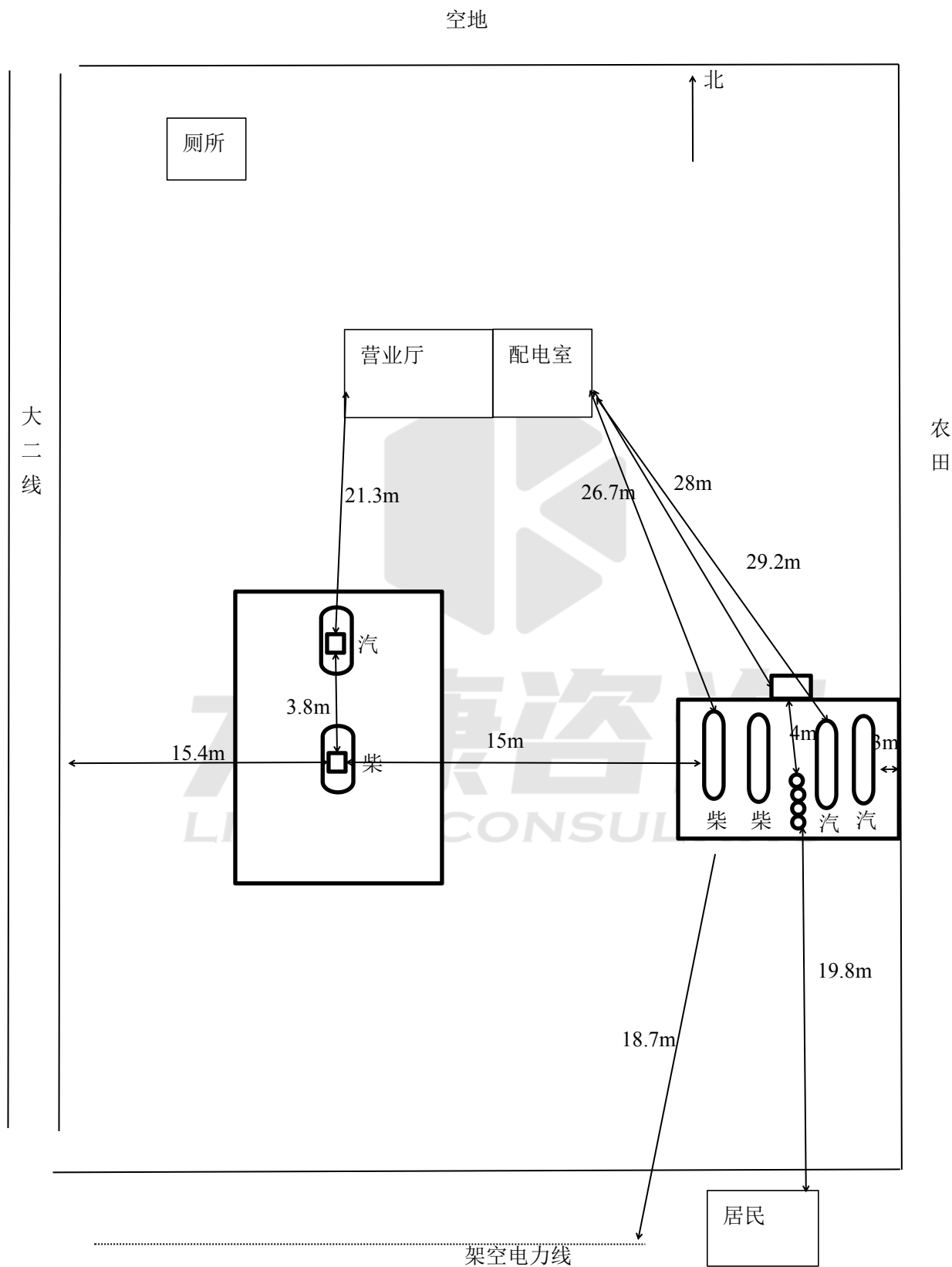
图 2.3-1 周边环境及总平面示意图
