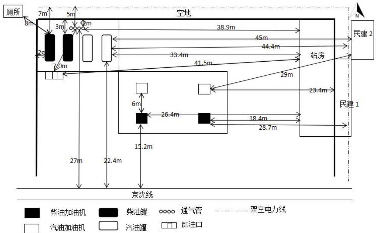
图 2.3-1 周边环境及总平面布置图
