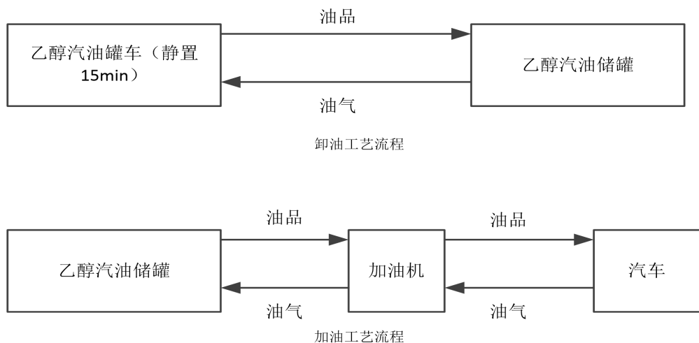
图 2.6-1 车用乙醇汽油工艺流程框图
