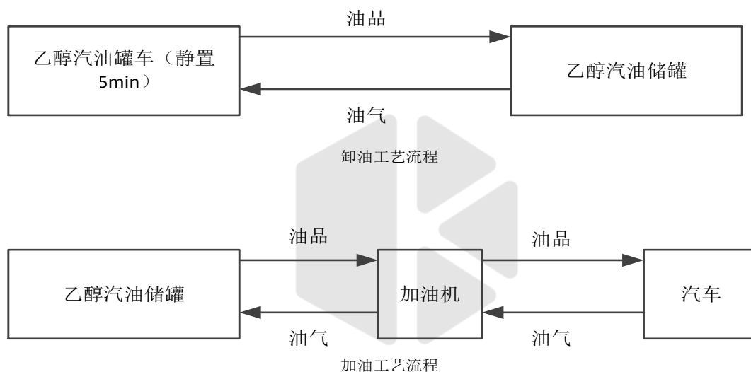
图 2.6-1 车用乙醇汽油卸油、加油工艺流程框图
