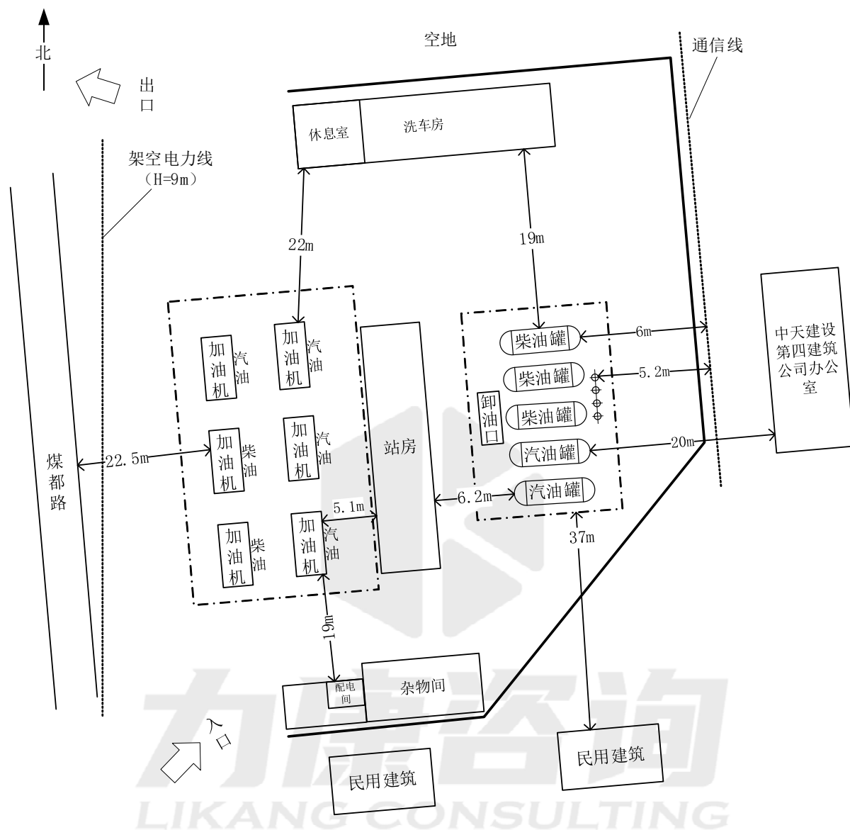
图 2.3-1 加油站总平面布置示意图
