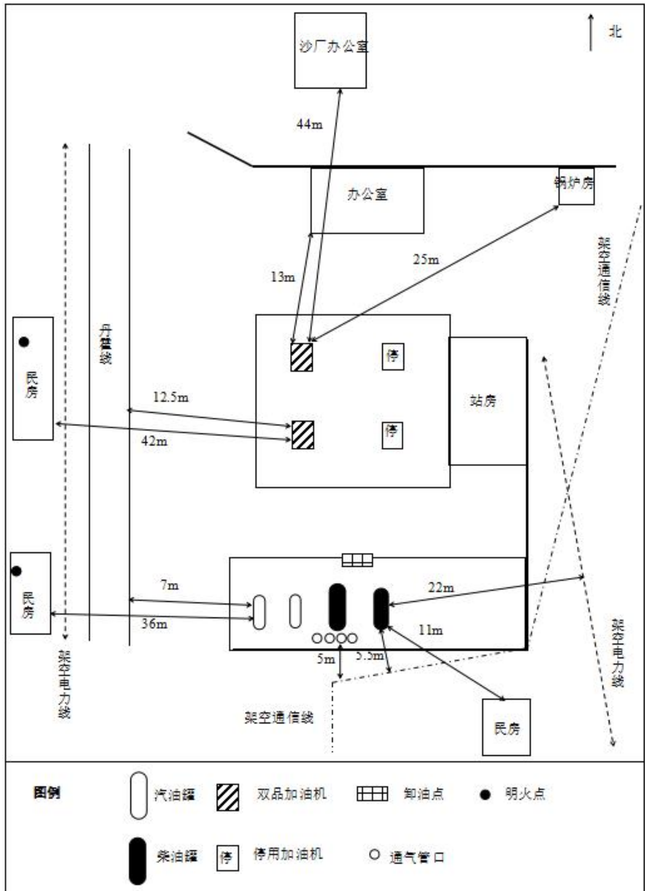
图 2.3-1 周边关系及总平面布置图
