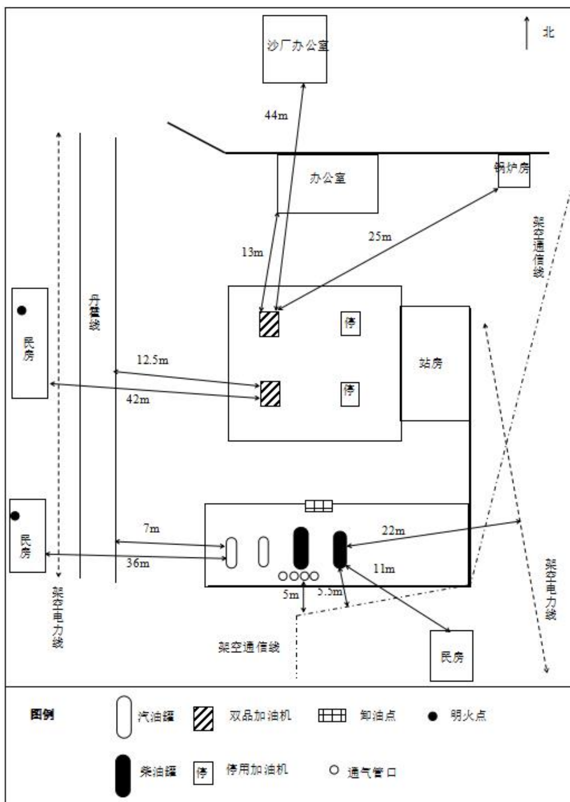
周边关系图及总平面布置图
