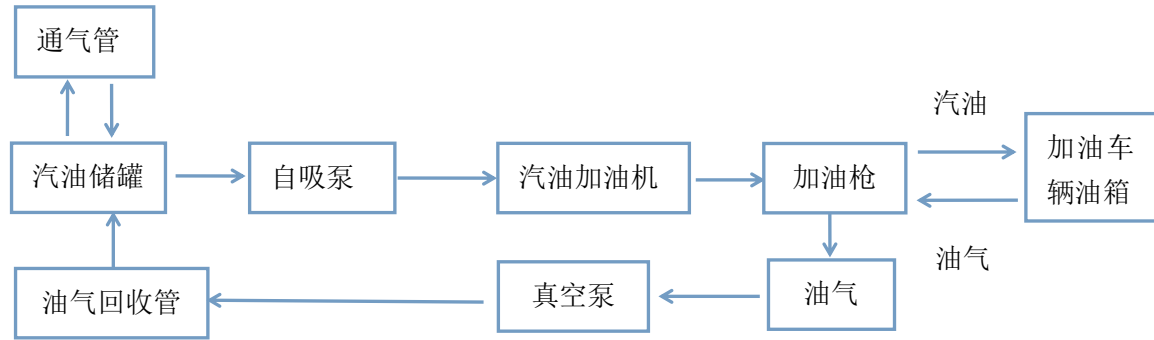
图 2.6-2 汽油加油工艺流程示意图
