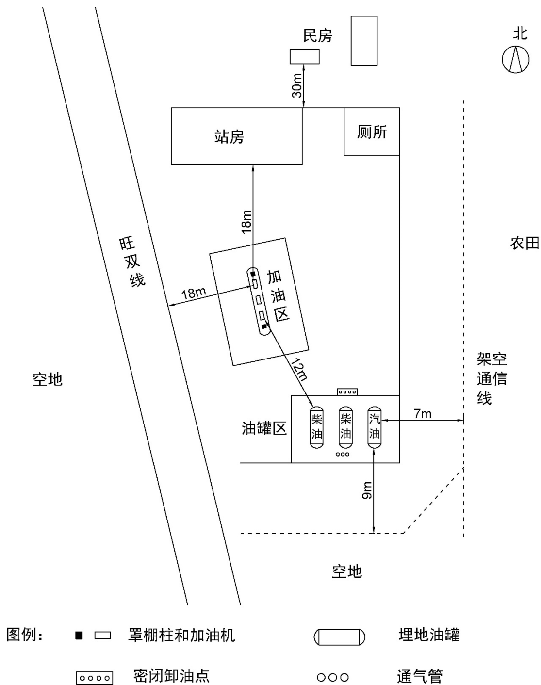
图 2.3-1 加油站总平面布置示意图
