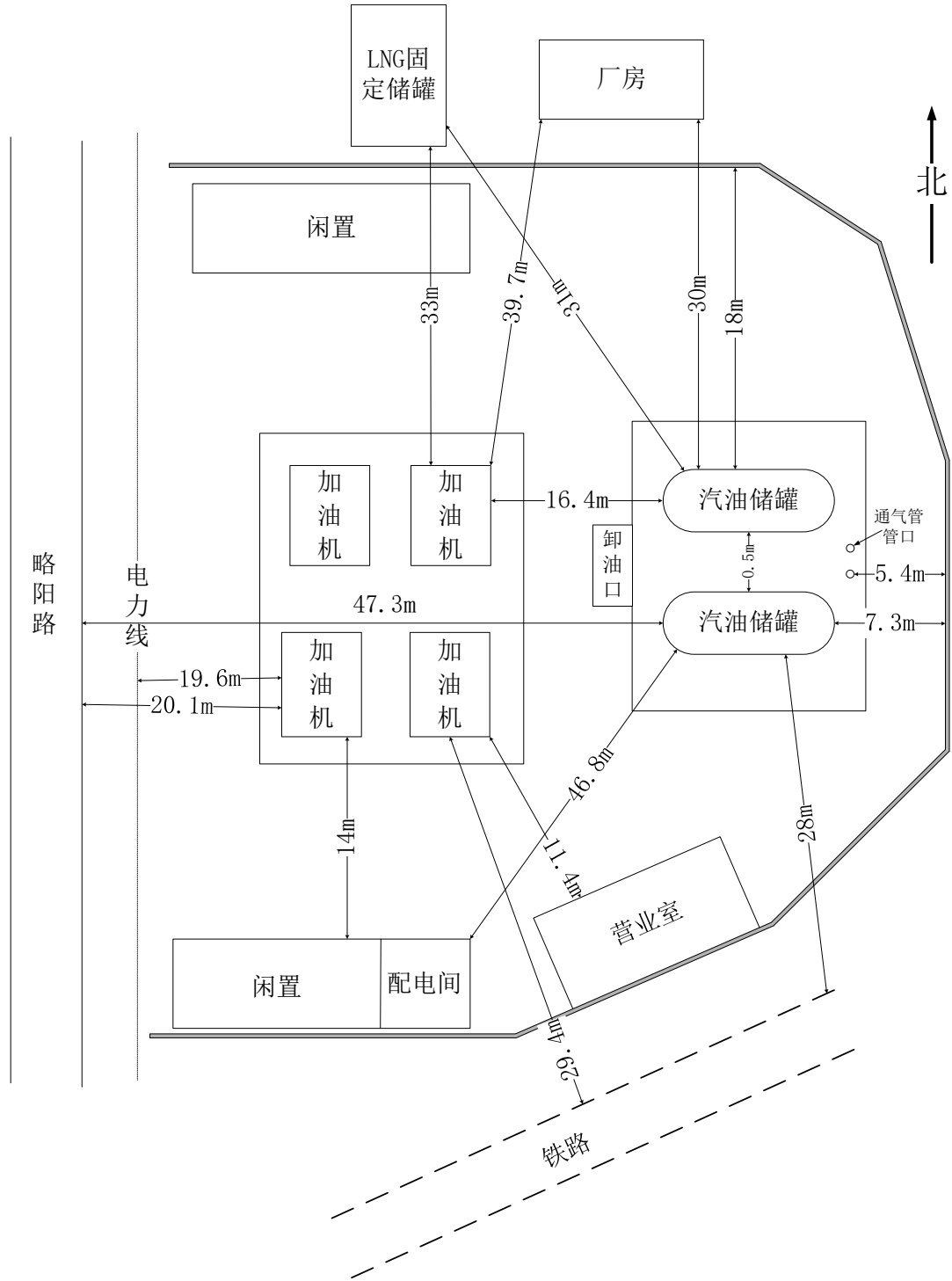
图 2.3-1 加油站周边环境和总平面布置示意图
