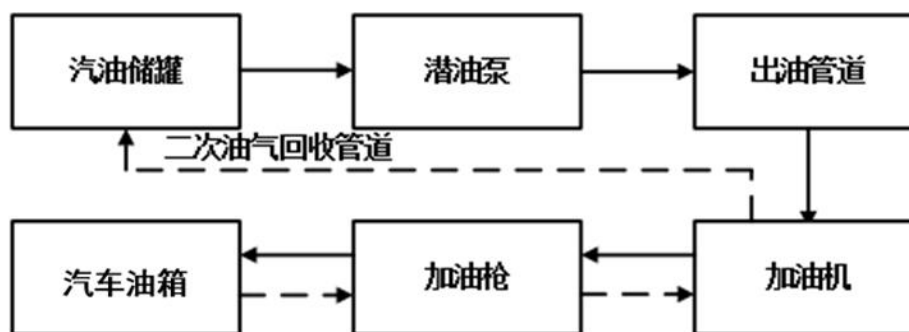
图 2.6-2 汽油加油流程图
