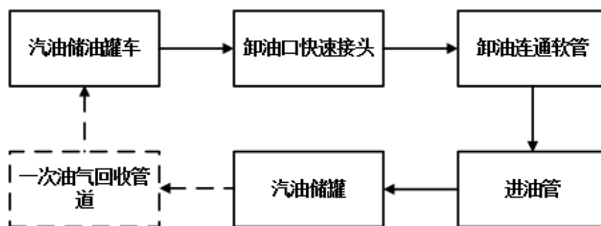
图 2.6-1 汽油卸油流程图
